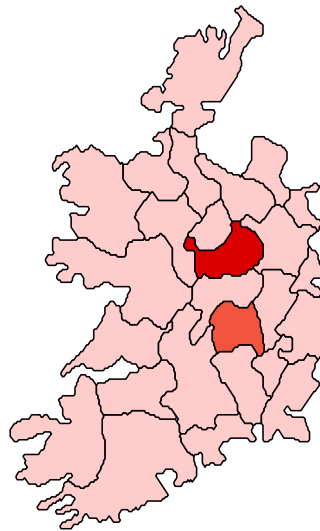
Fig.5.11. P-Values for G
