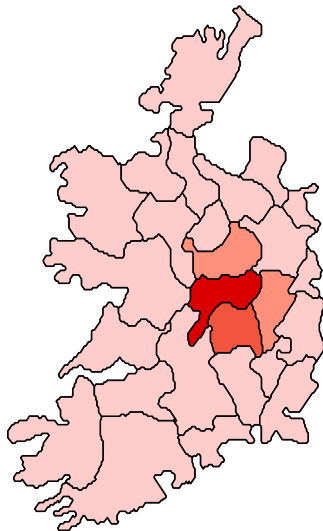
Fig.5.10. P-Values for G^*
